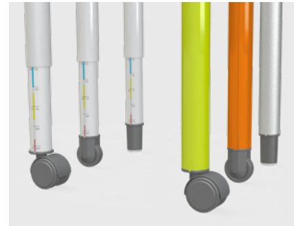
Modulares Fußkonzept (Lenkrolle, Bockrolle, TPE-Gleiter) mit oder ohne Höhenverstellung (in 30 mm Rastern).
