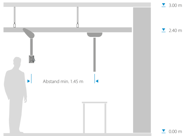
Schnitt
