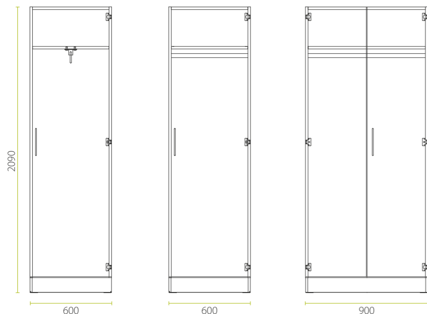
Garderobenschrank mit Garderobenzug
